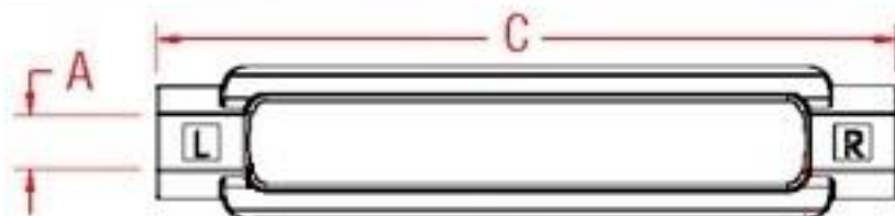
Рисунок 1. Чертеж тела талрепа.
